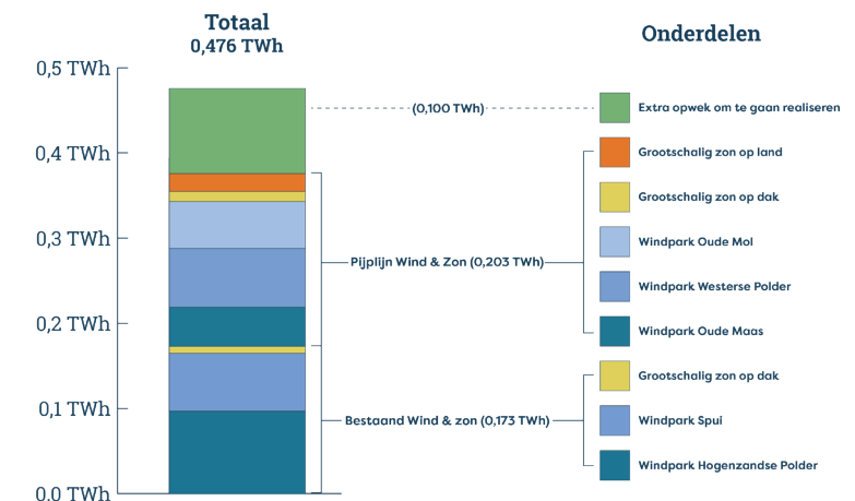
Figuur 1: Bijdrage van de regio Hoeksche Waard aan nationale doelstellingen van 35 TWh hernieuwbare elektriciteit (bandbreedte 0,376 - 0,476 TWh)
