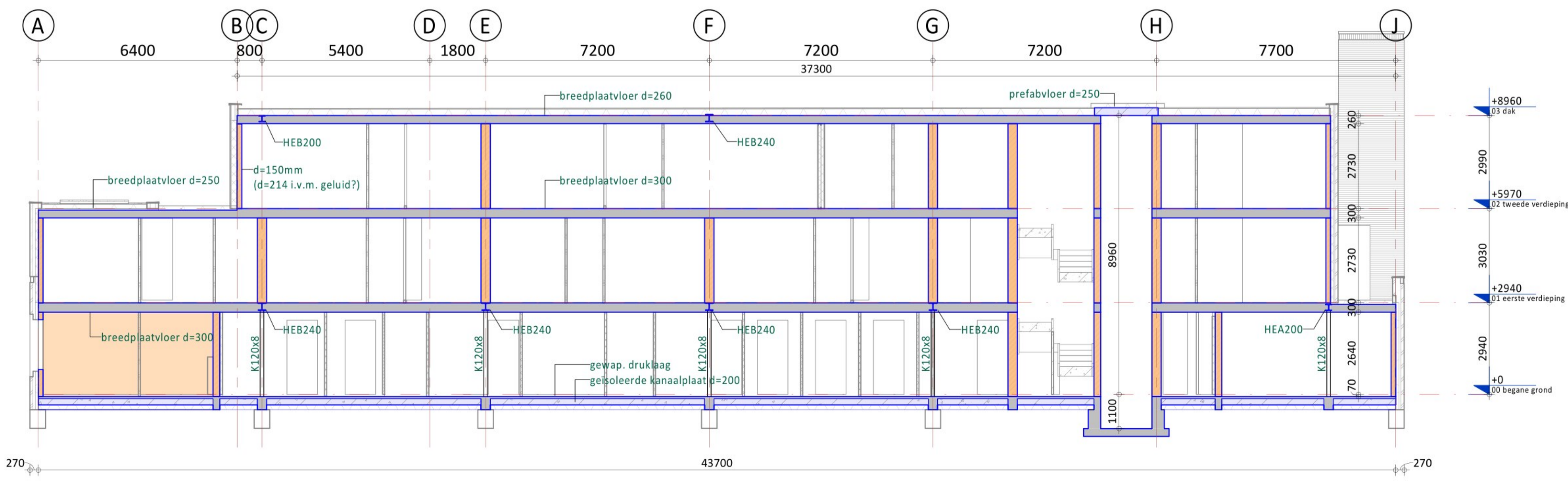
Drasn. G-G
