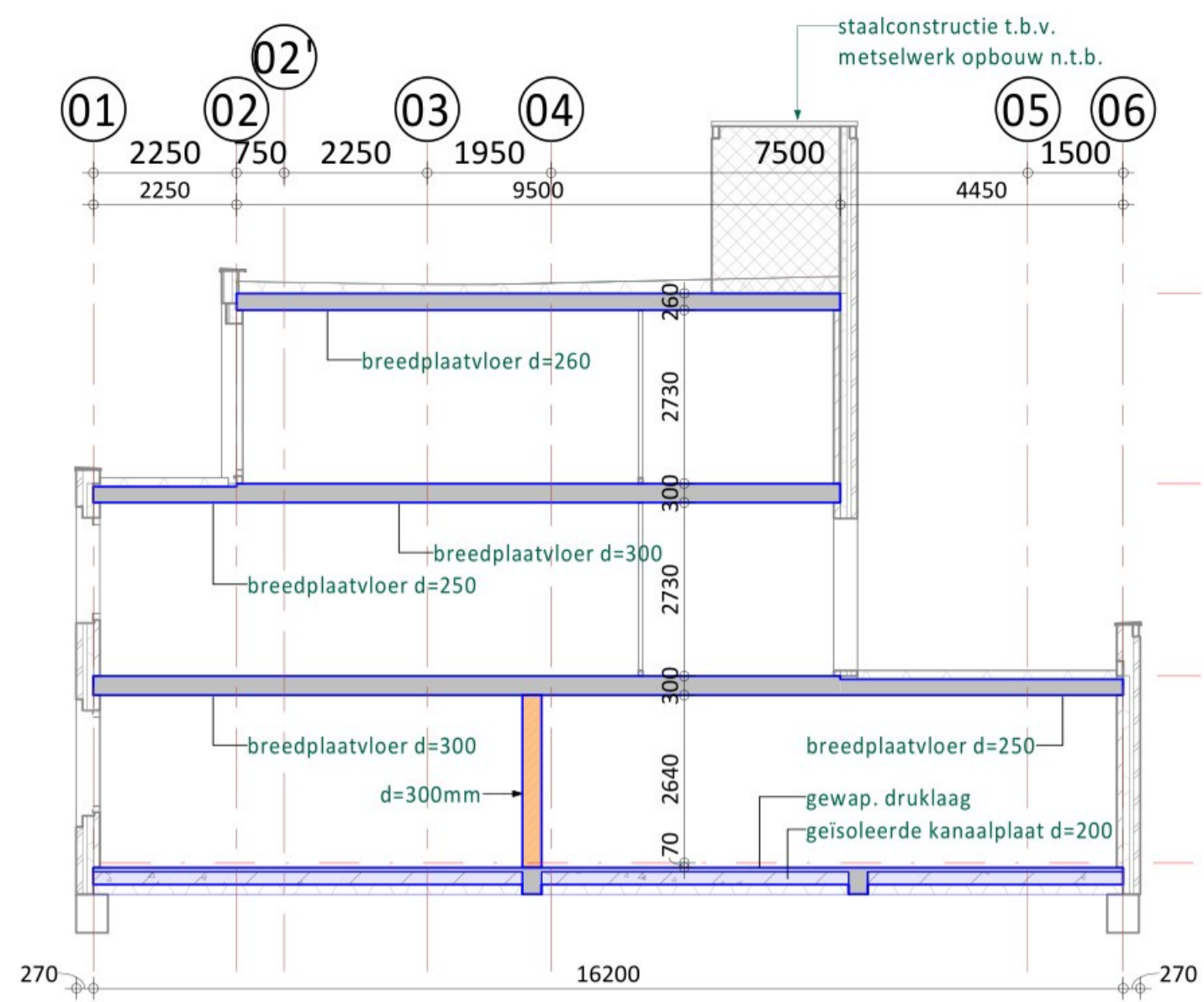
Drasn. A-A
