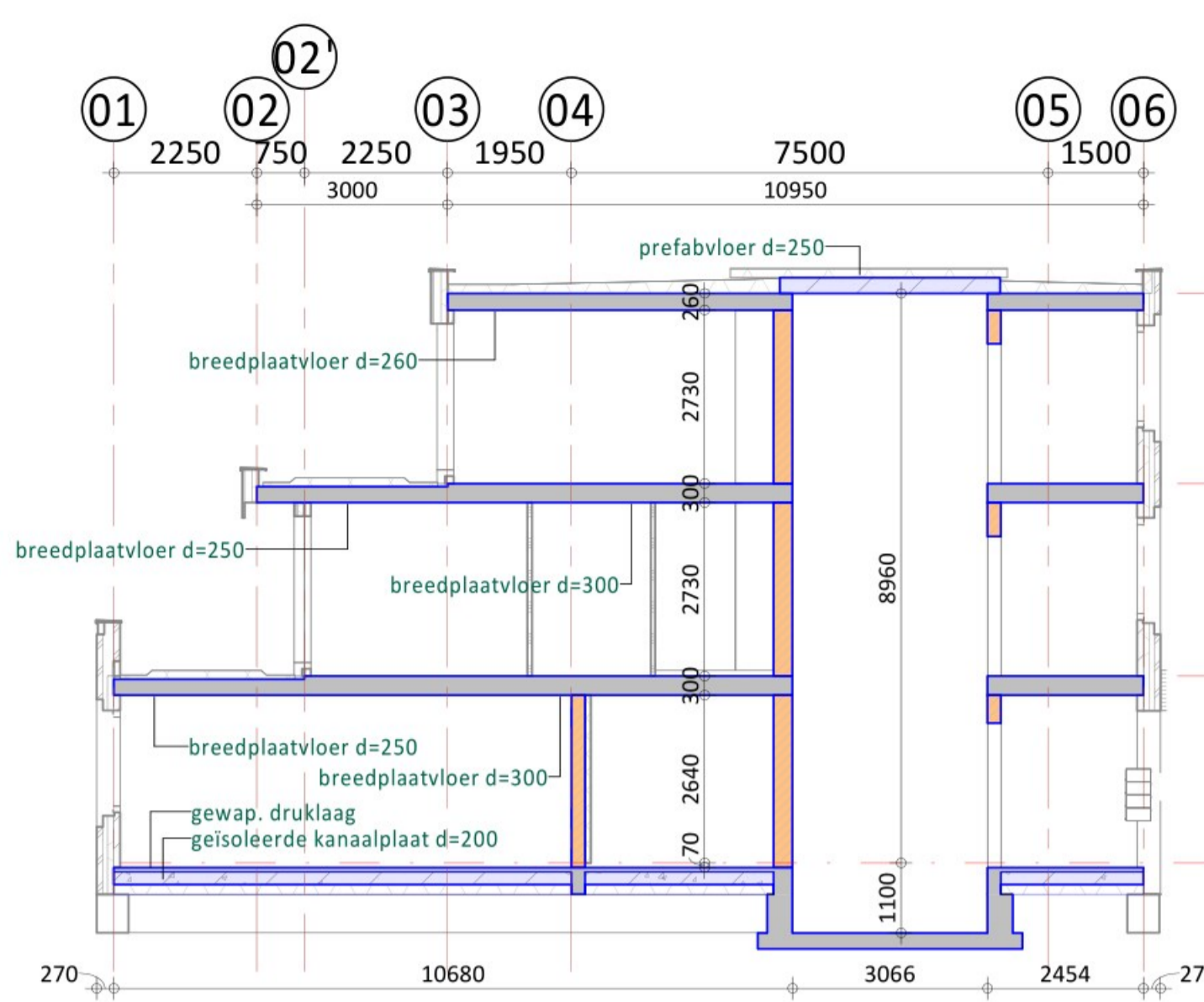
Drasn. B-B
