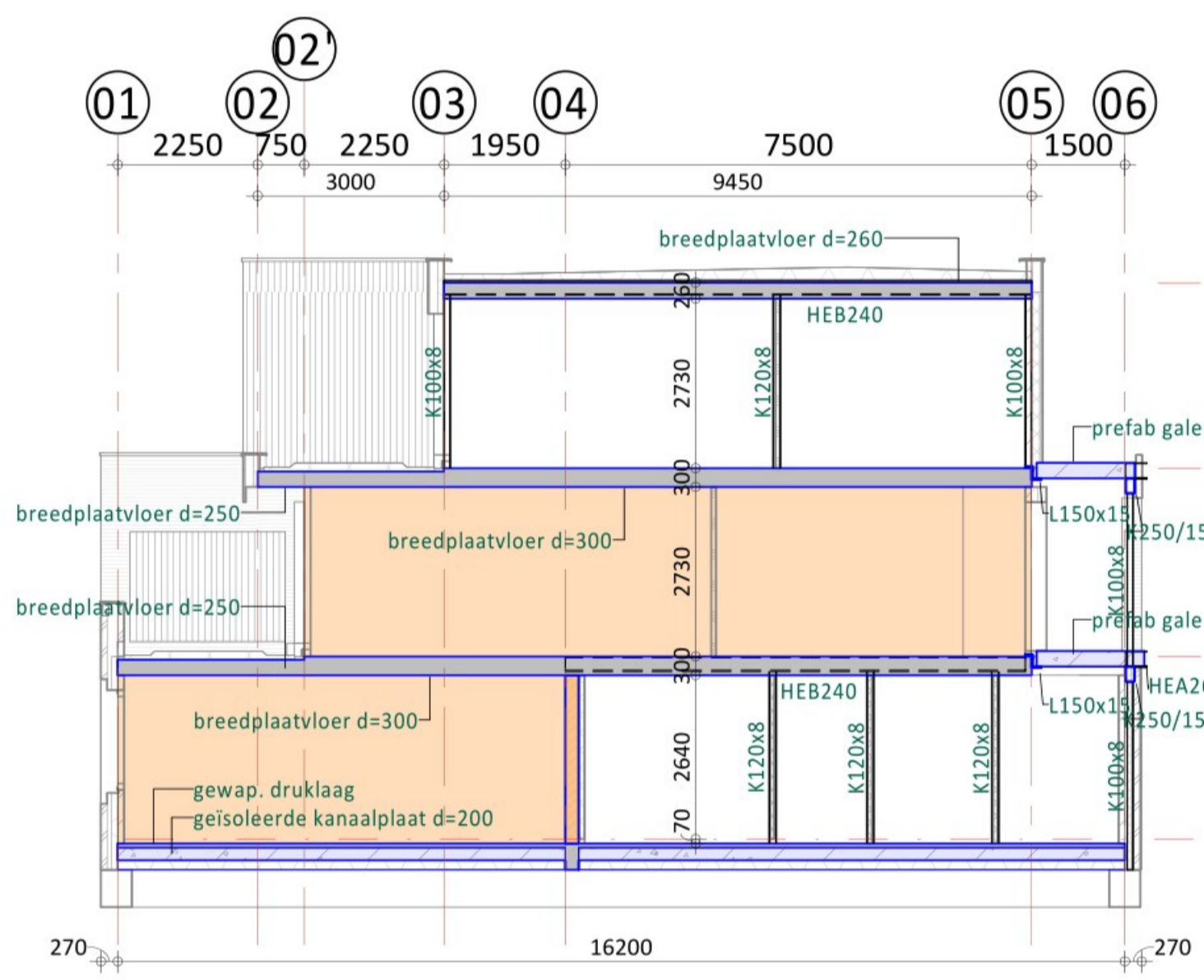
Drasn. D-D
