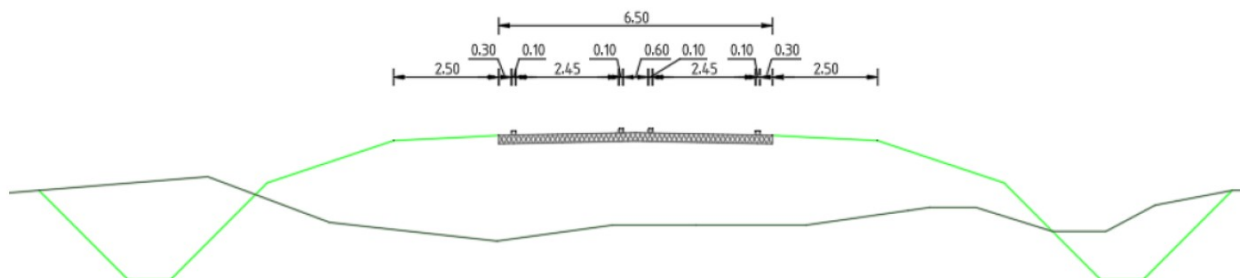
Figuur 3.2 Principeprofiel GOW60
