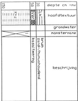
Boorprofiel nr. 63
