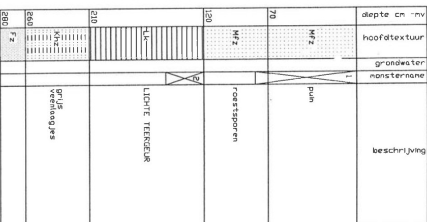
Boorprofiel nr. 74
