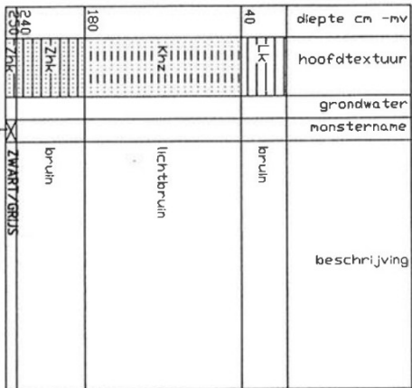
Boorprofiel nr. 64
