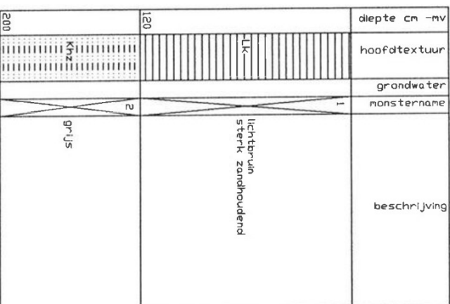
Boorprofiel nr. 73
