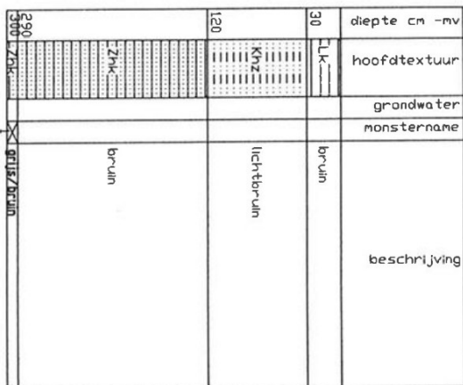
Boorprofiel nr. 65
