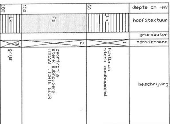
Boorprofiel nr. 72
