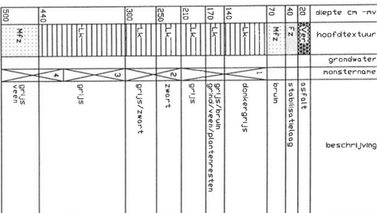
Boorprofiel nr. 66
